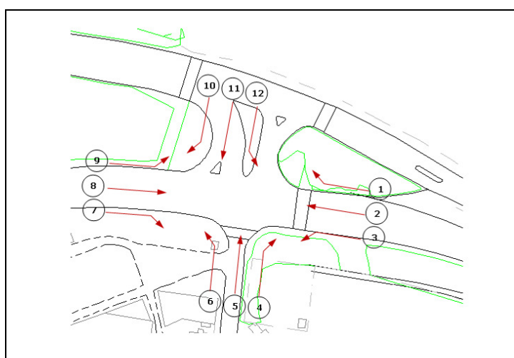
Figura 106 – Numeração dos movimentos no posto de contagem nº 1
