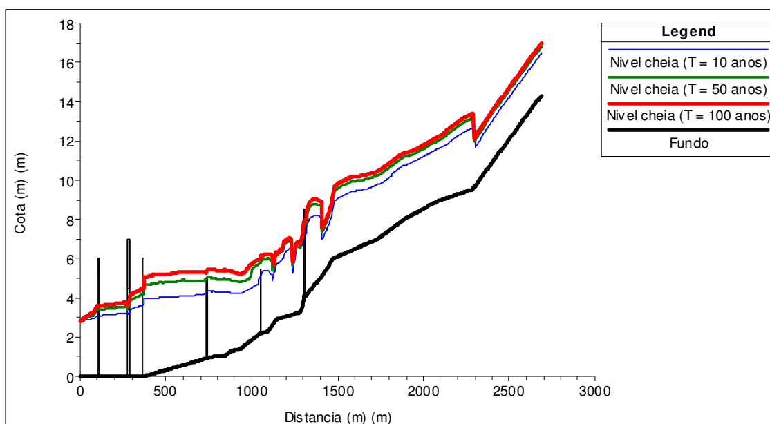
Figura 50 – Perfis longitudinais dos níveis da superfície livre obtidos com HEC-RAS
