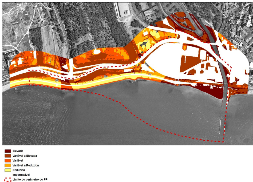
Figura 39- Susceptibilidade à erosão hídrica (Fonte: GEOTPU, 2010)
