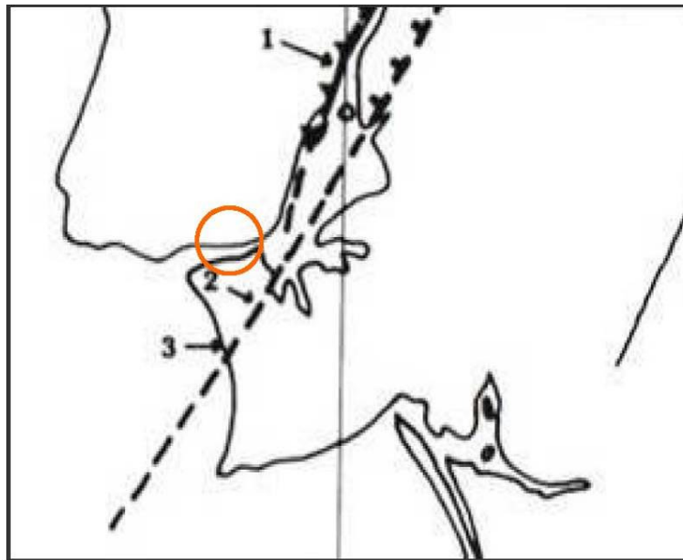
Figura 36 – Extracto da Carta Neotectónica simplificada de Portugal Continental (Fonte: CABRAL, 1995)
