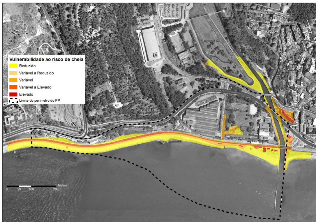
Figura 74 – Áreas susceptíveis à inundaç o de origem marinha e fluvial (Fonte: GEOTPU, 2010)
