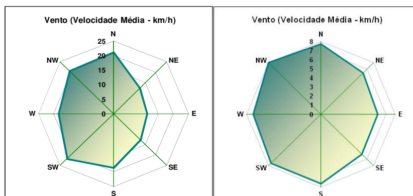
Figura 30 - Diagrama da velocidade do vento (km/h) para as Estações Meteorológicas de Lisboa/Tabada da Ajuda e Lisboa/Aeroporto da Portela (Fonte: INMG, 1991)
