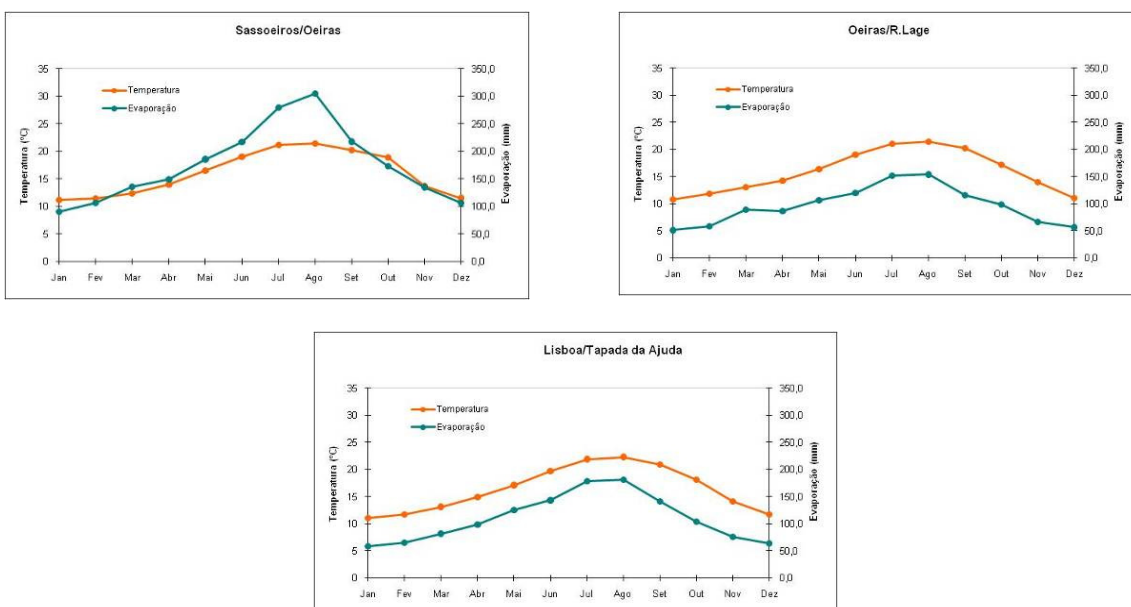
Figura 27 – Evaporação versus temperatura para as Estações Meteorológicas de Sassoeiros/Oeiras, Oeiras/R. Lage e Lisboa/Tapada da Ajuda (Fonte: INMG, 1991)
