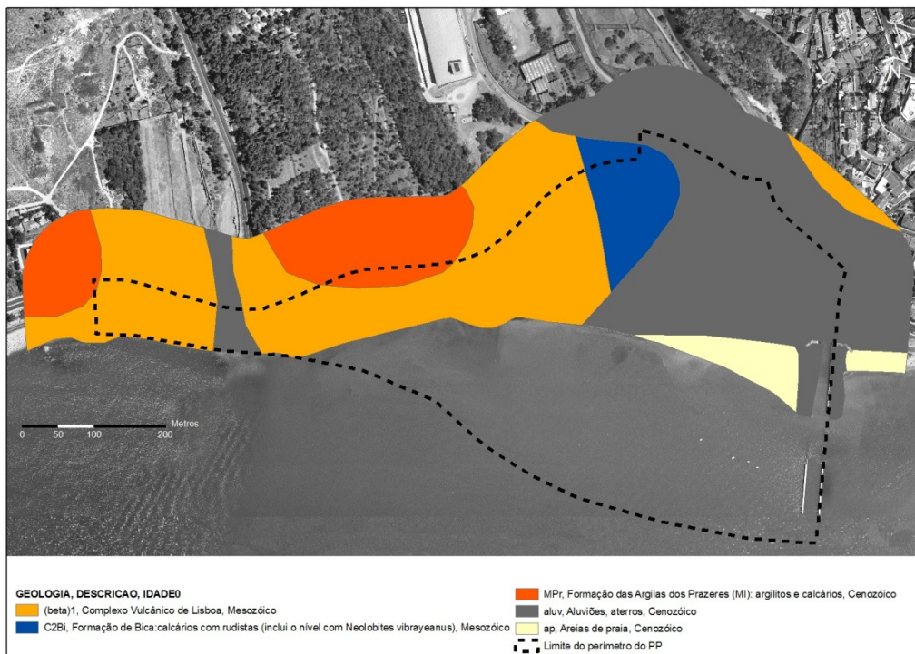
Figura 35 - Litologia da área de intervenção do Plano de Pormenor de Porto Cruz (Fonte: GEOTPU, 2010)
