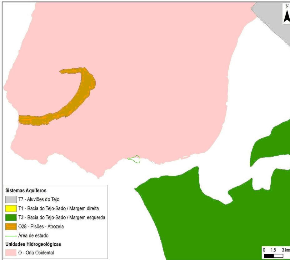
Figura 56 – Unidades hidrogeológicas (Fonte: INAG)
