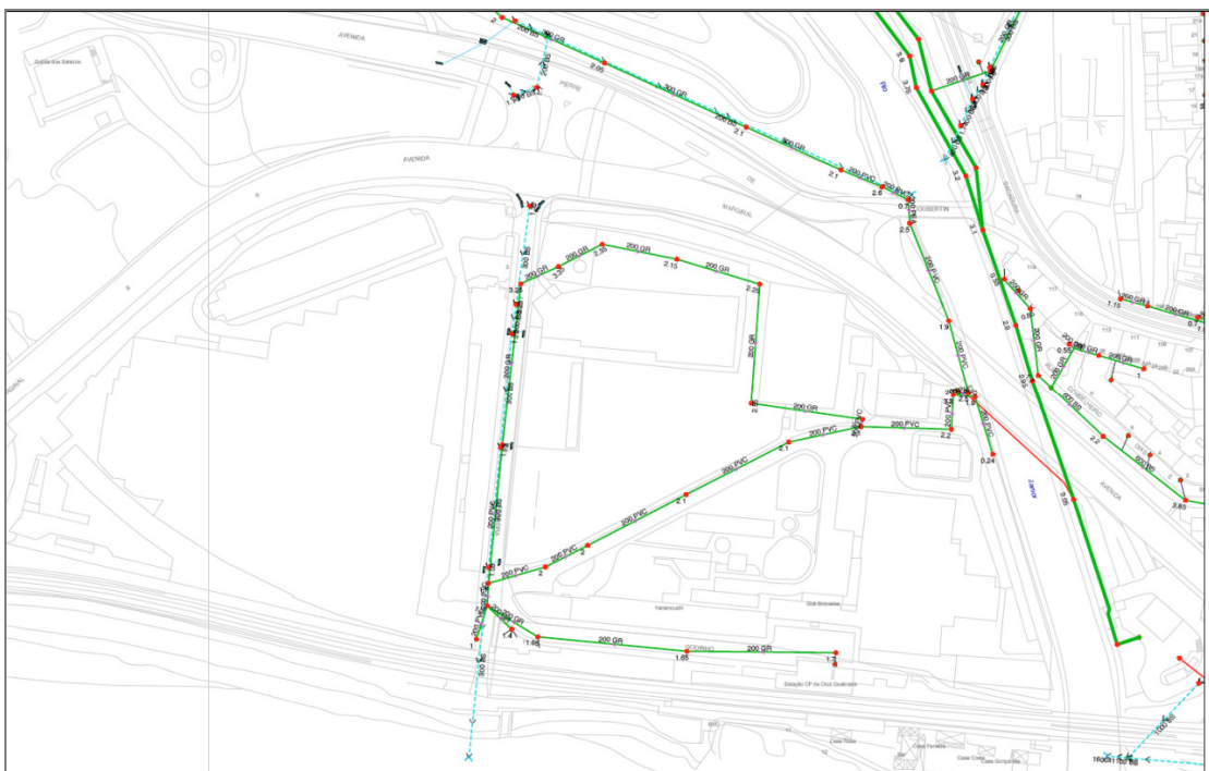
Figura 97 – Rede de drenagem de águas residuais (Fonte: SMAS Oeiras e Amadora)
